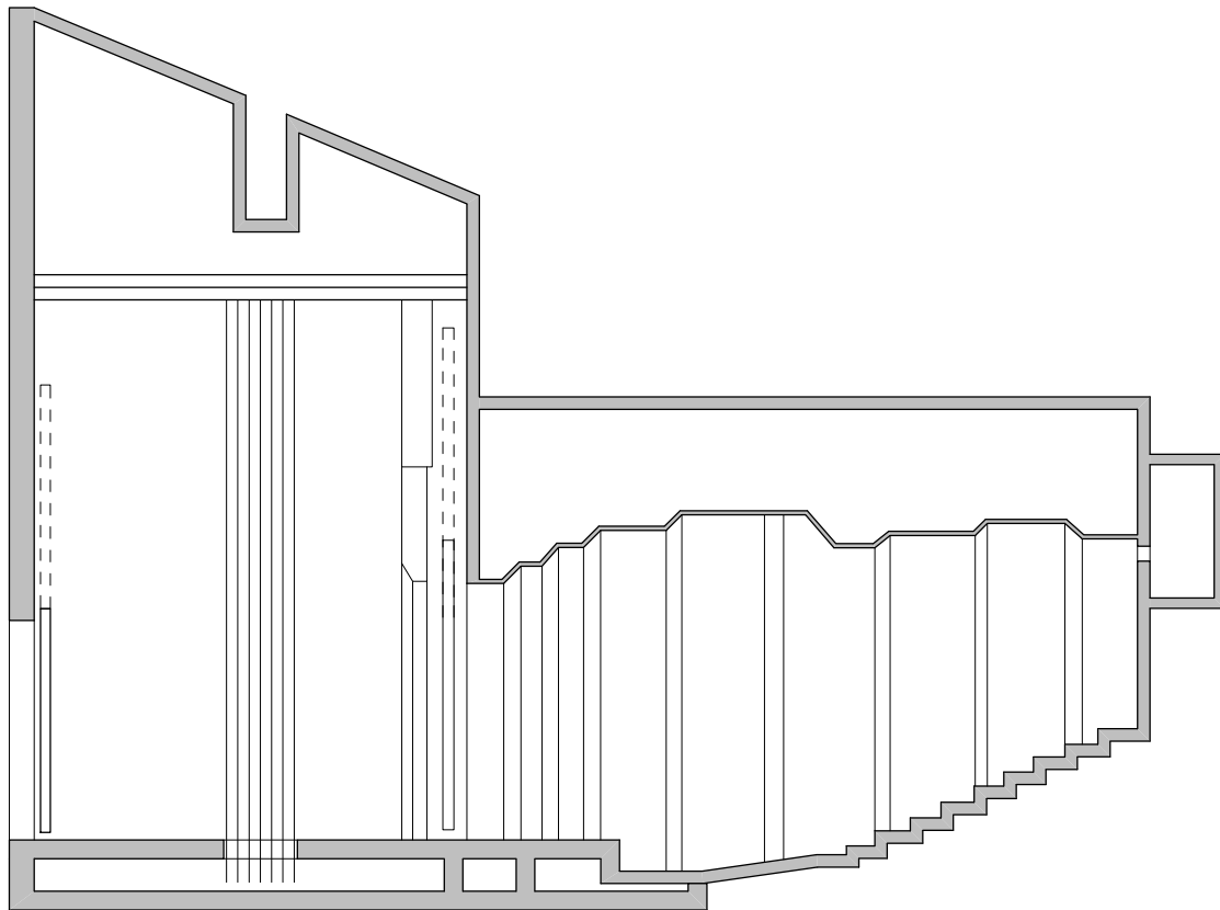
Pozorište u Pirotu presek R 1:200
