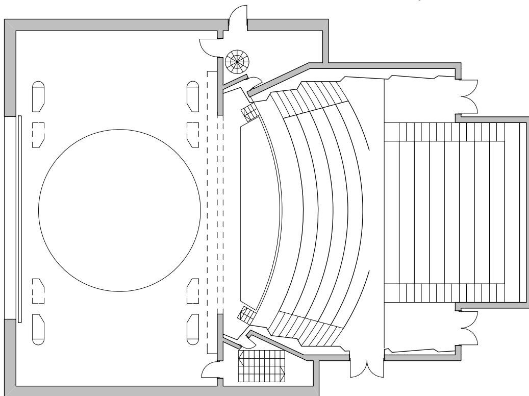
Pozorište u Pirotu osnova R 1:200
